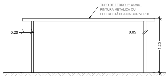
EQ. 01 BARRAS PARALELAS ELEVAÇÃO Escala -----1:50
