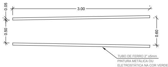
EQ. 01 BARRAS PARALELAS VISTA SUPERIOR Escala -----1:50
